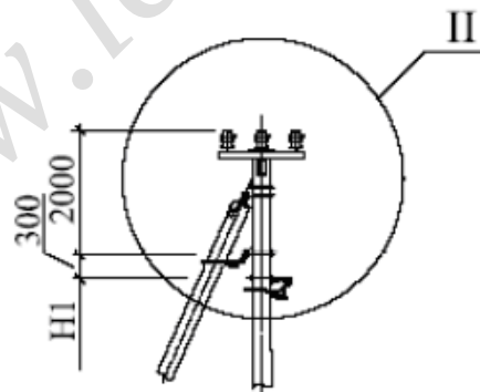
Stūra atgāžņstarpbalsts SSs20.I-HT-04Pn (pārējo skatīt stūra atgāžņstarpbalstu SSs20.I-HT-04Ps)
