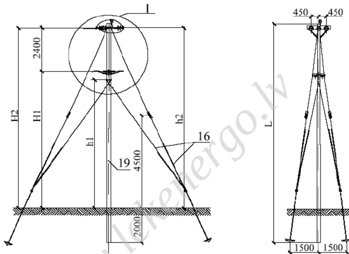
Atsaišenkurbalsts Ea20.I-HP-04Ps
