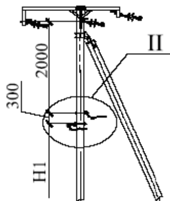
Stūra atgāžņstarpbalsts SSs20.I-HP-04Pn (pārējo skatīt stūra atgāžņstarpbalstu SSs20.I-HP-04Ps)
