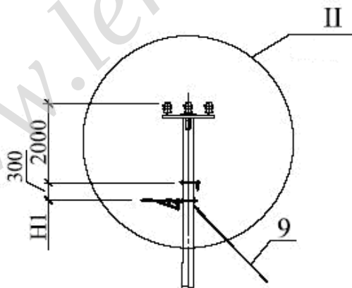
Nozarojuma atsaišstarpbalsts NSa20.I-HT-04Ps
