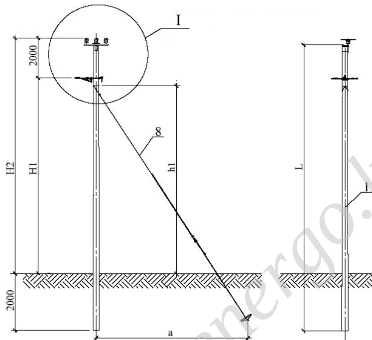
Nozarojuma atsaišstarpbalsts NSa20.I-HT-04Ps
