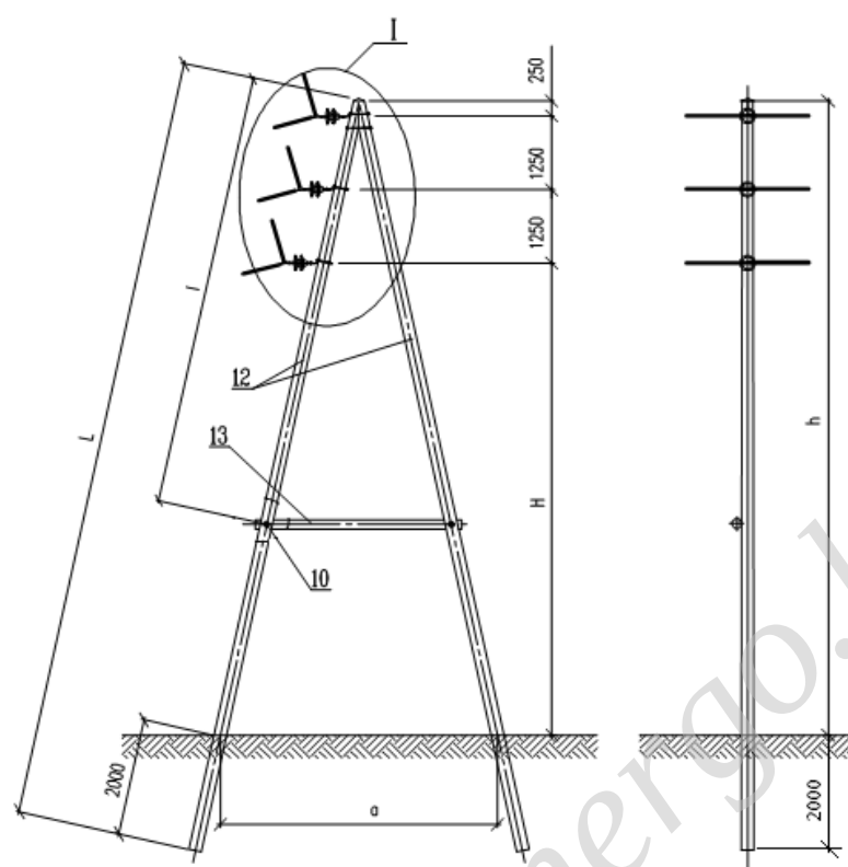
Balsta uzstādīšanas shēma
